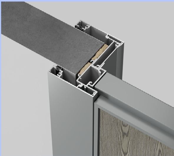
Короб Integral Reverse (44) обратное открывание
