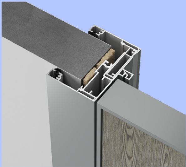
Короб Integral (44) прямое открывание
