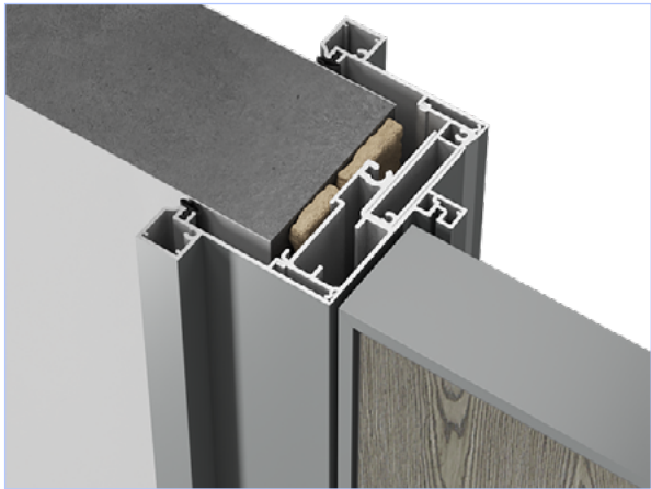
Наличник объемный (70)
