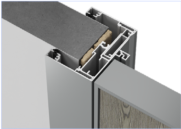
Наличник прямой (70)
