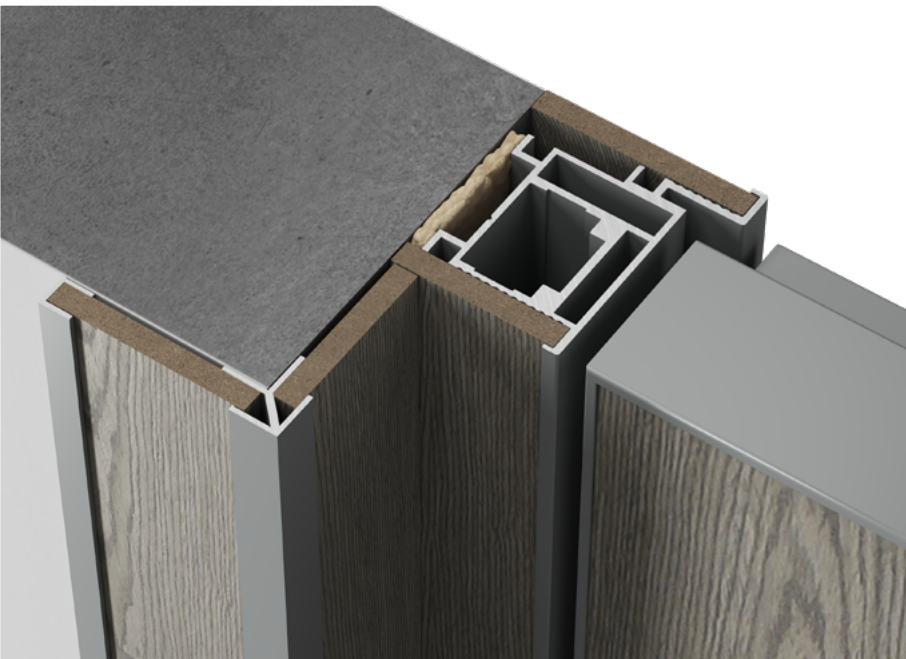
Виды облицовочных алюминиевых профилей
