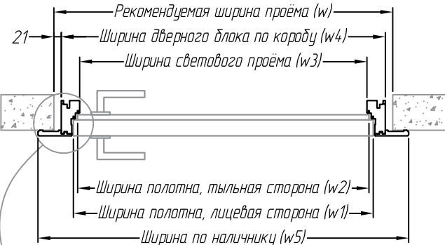
Соотношение параметров дверного блока и проёма по ширине, мм
