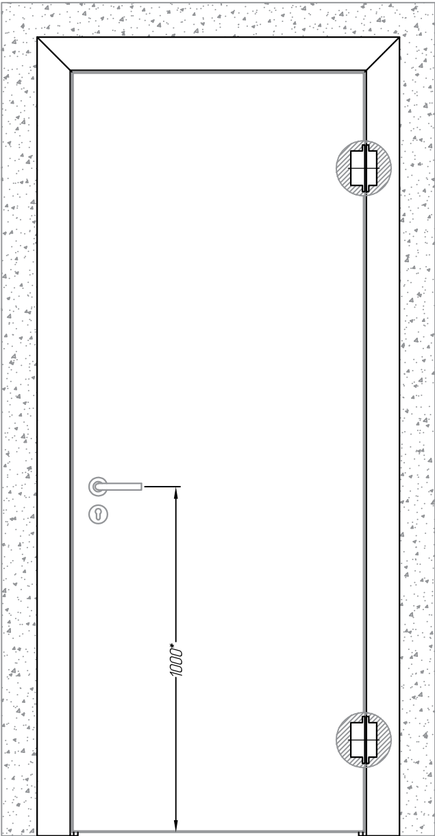
Соотношение параметров дверного блока и проёма по высоте, мм
